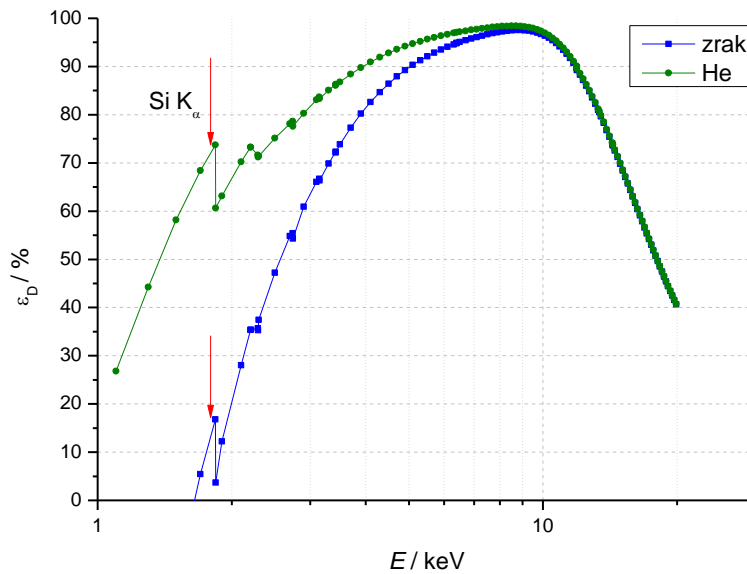
Slika 3.5. Efikasnosti X-123SDD detektora u ovisnosti o energijama karakterističnih x-zraka koje prolaze kroz zrak 84 ili kroz helij 85
