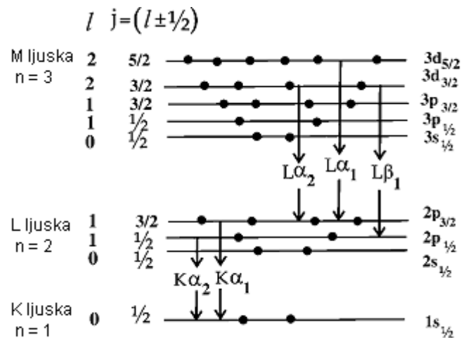
Slika 3.11. Dozvoljeni elektronski prijelazi u ljuskama [98]
