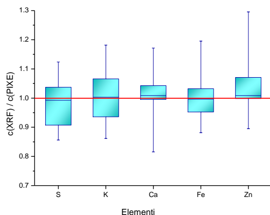
Slika 6.16. Box-whisker plot omjera XRF i PIXE koncentracija glavnih elemenata za uzorke prikupljene u Luka Rijeka od 6. 8. 2013. do 28. 2. 2014. godine
