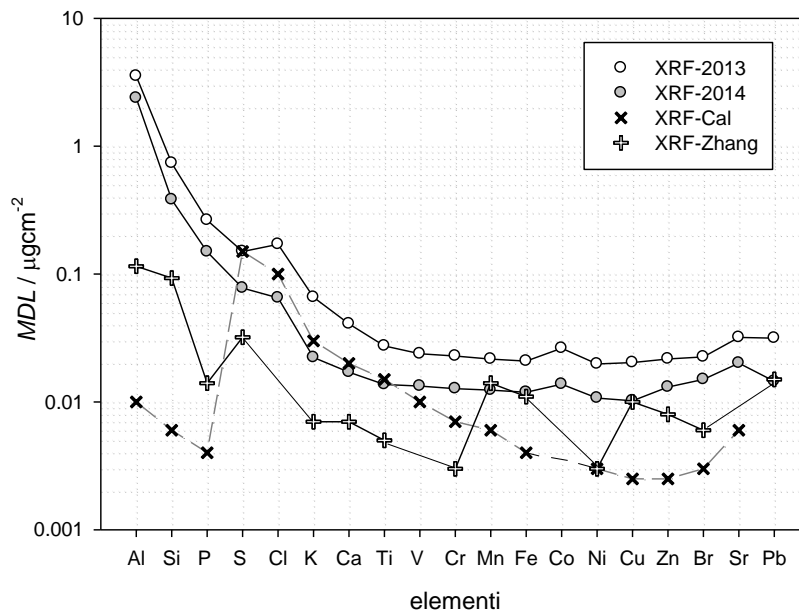
Slika 6.2. Usporedba prosječnih donjih granica detekcije (MDL) elemenata od Al do Pb na teflonskim filtrima dobivenih pomoću XRF tehnika u Rijeci (XRF-2013, XRF-2014), Italiji (XRF-Cal) i Kini (XRF-Zang)
