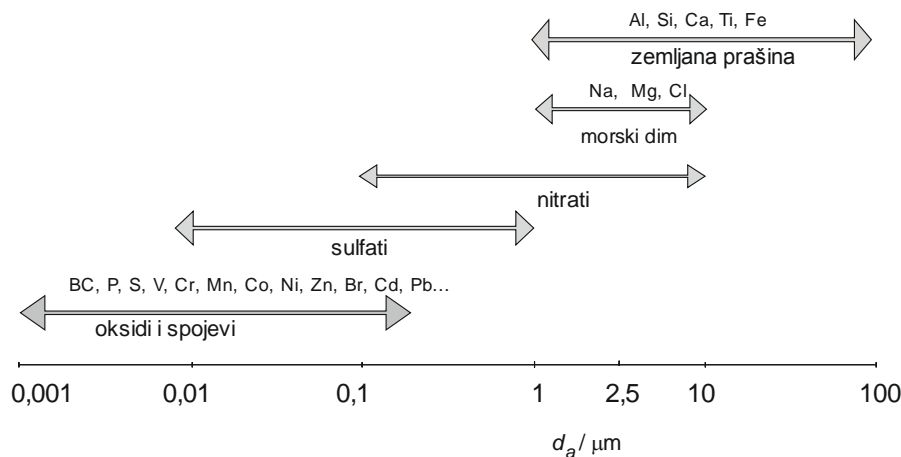
Slika 2.5. Aerosoli prirodnog i umjetnog porijekla prikazani prema aerodinamičkom promjeru
