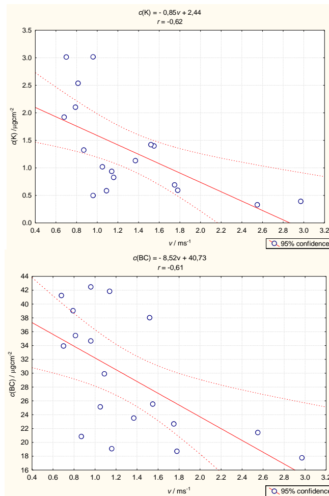
Slika 6.8. Dijagrami raspšenja izmjerenih koncentracija K i BC s brzinama vjetra
