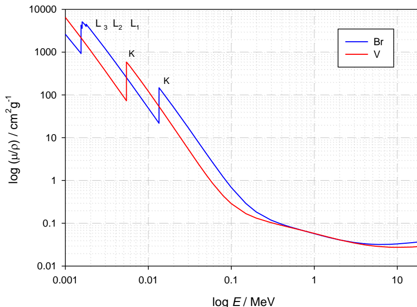
Slika 3.14. Maseni koeficijenti prigušenja Br i V u ovisnosti o energiji fotona
