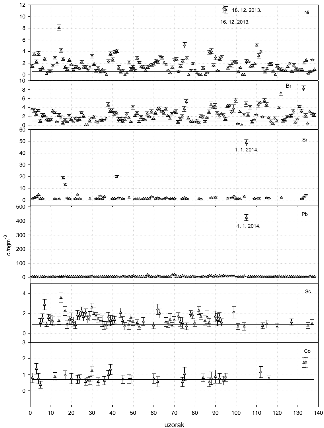
Slika 6.20. Trend promjena XRF koncentracija s ukupnim pogreškama i MDL-ovima u \text{ngm}^{-3} elementa u tragovima za uzorke prikupljene od 6. 8. 2013. do 28. 2. 2014. godine
