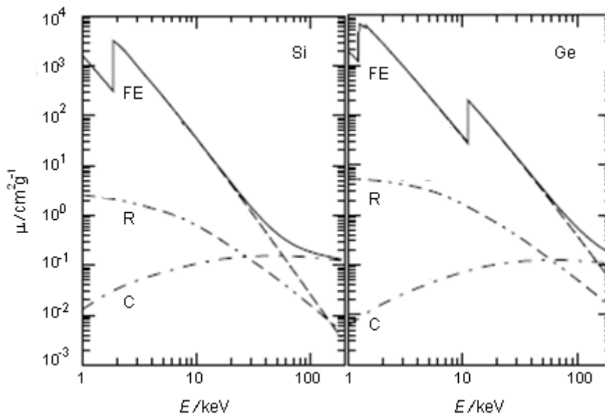
Slika 3.12. Maseni koeficijenti prigušenja Si i Ge u ovisnosti o energijama fotona. Oznake: FE - fotoelektrični efekt, R - Rayleighijevo raspršenje, C - Comptonovo raspršenje [6]
