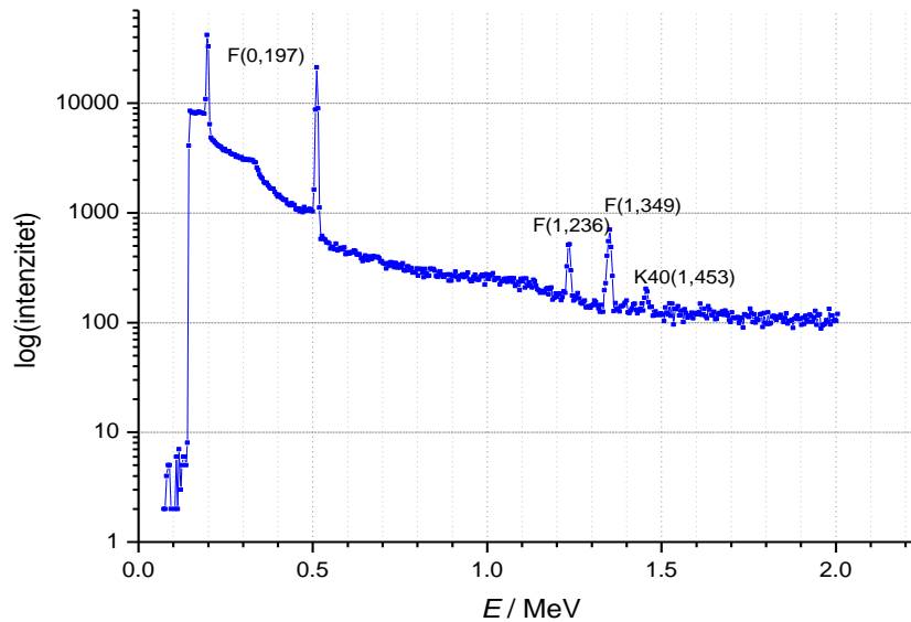
Slika 3.19. Spektar aerosola iz Trpimirove ulice uzorkovan 24./25. veljače 2012. godine dobiven pomoću PIGE tehnike. Korištena je energija protona od 2,6 MeV i struja od 12 nA proizvedena pomoću 3 MV Tandem Van de Graff te je prikupljen naboj 3 \mu C.
