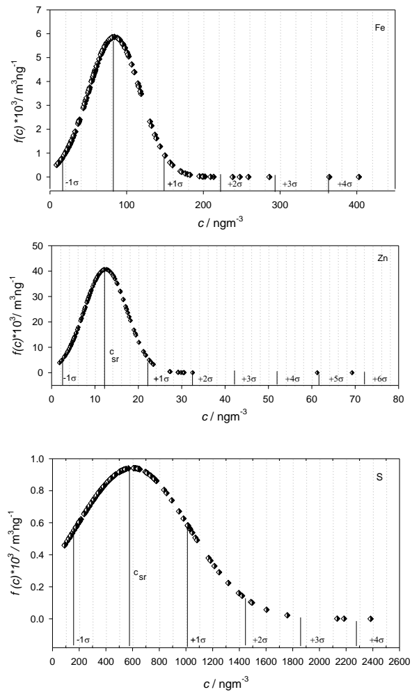
Slika 4.3. Pozitivno asimetrična distribucija izmjerenih koncentracija Fe, Zn i S u finoj frakciji aerosola uzorkovanoj u području „Luka Rijeka“ od 6. kolovoza 2013. do 28. veljače 2014. godine
