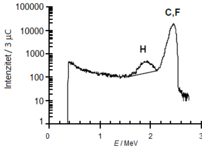
Slika 3.18. Primjer PESA spektra aerosola [24]
