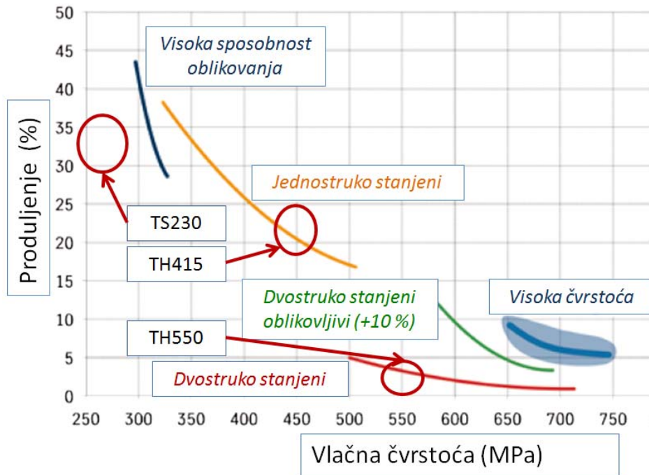
Slika 3.6 Tankostjeni materijali, odnos produljenja i vlačne čvrstoće [66]
