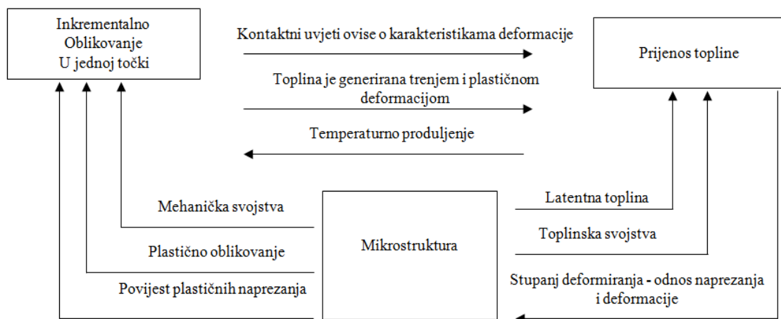
Slika 2.19 Interakcija parametara u procesu plastičnog oblikovanja [50]
