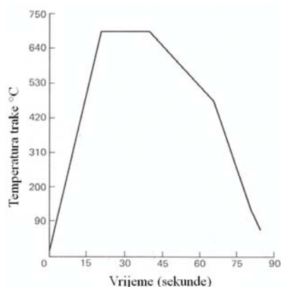
Slika 3.4 Vrijeme trajanja kontinuiranog žarenja (CA) [19]
