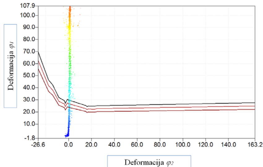
Slika 9.13 Dijagram sposobnosti oblikovanja za materijal TS230, kut od 58°, visina 25 mm
