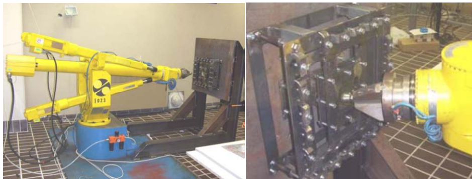
slika 2.7 Upotreba robota u SPIF procesu [28]
