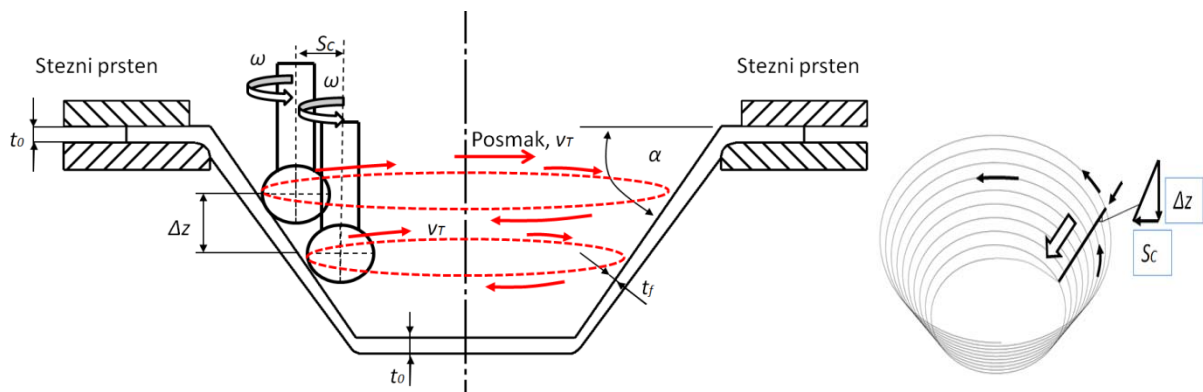
Slika 2.1 Shema inkrementalnog oblikovanja krnjeg stošca u jednoj točki, poprečni presjek - lijevo, spiralna putanja vertikalnog pomaka \Delta z i S_C - desno [23]
